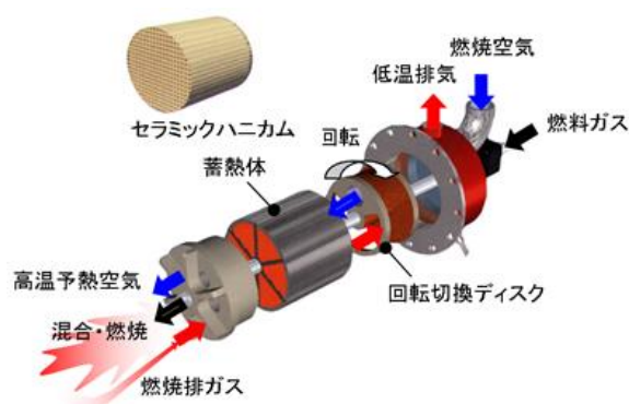
イラスト リジェネバーナの構造
