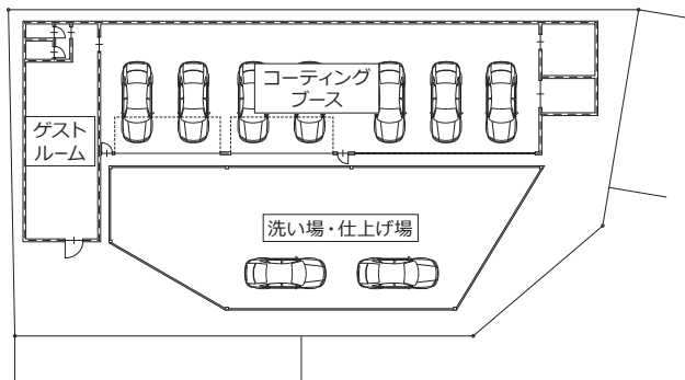
【店舗平面図】
