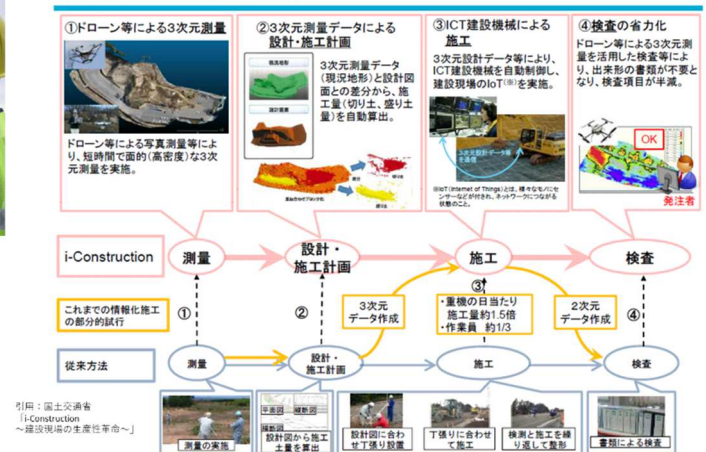
（参考）土木建築分野のDX例
