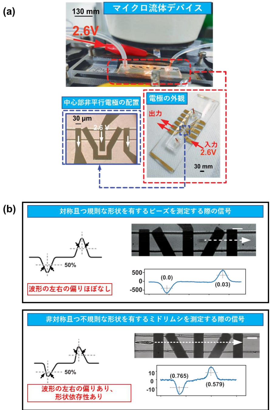
図2 ユーグレナの電気インピーダンス顕微観察システムとその原理
