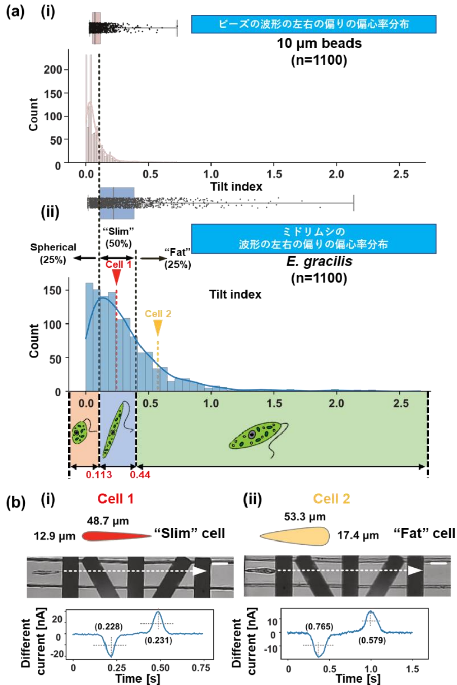
図3 1,100個のビーズとユーグレナのインピーダンス信号偏心率
