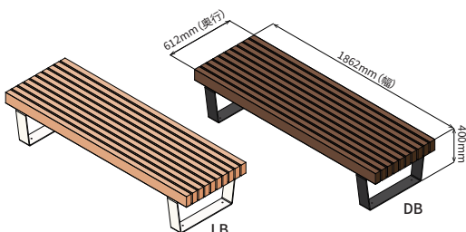
ライナスベンチ 0618 ¥180,000 (税抜定価) W1862 D612 H400 66kg
