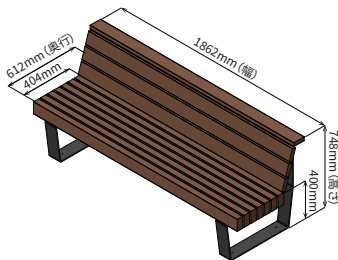
ルーシーベンチ 0618 DB
