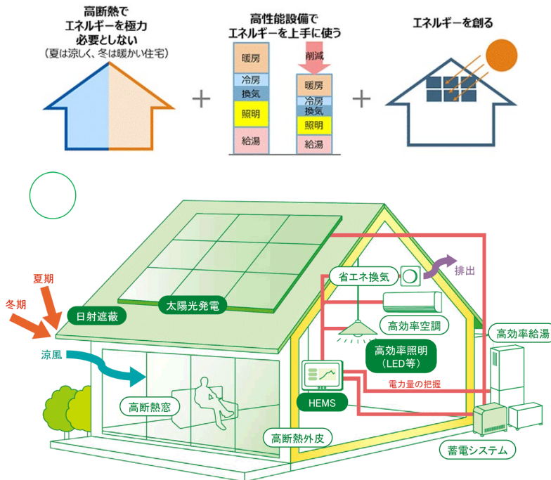
【図2】 ZEH（ネット・ゼロ・エネルギー・ハウス）のイメージ図
