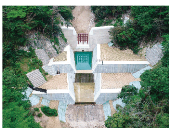
堰堤工事
