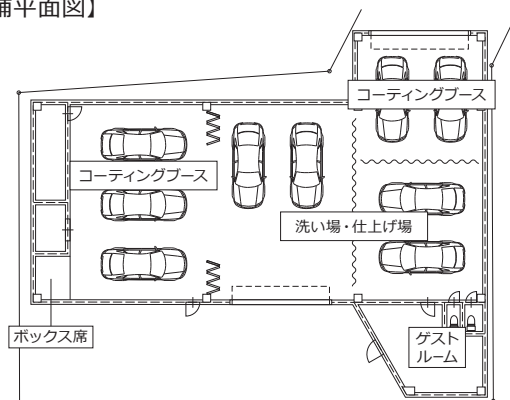
【店舗平面図】
