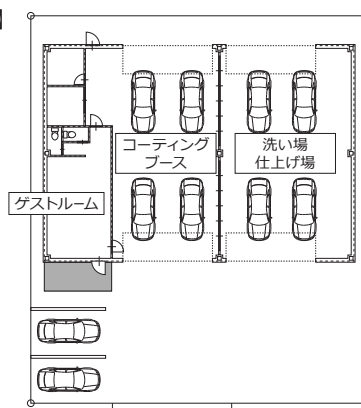
【店舗平面図】
