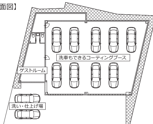
【店舗平面図】
