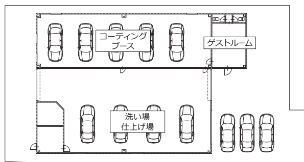
【店舗平面図】
