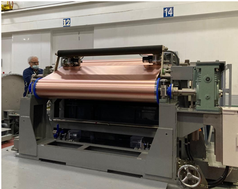
写真： 米国カムデン工場内に設置された車載電池用銅箔製造装置
