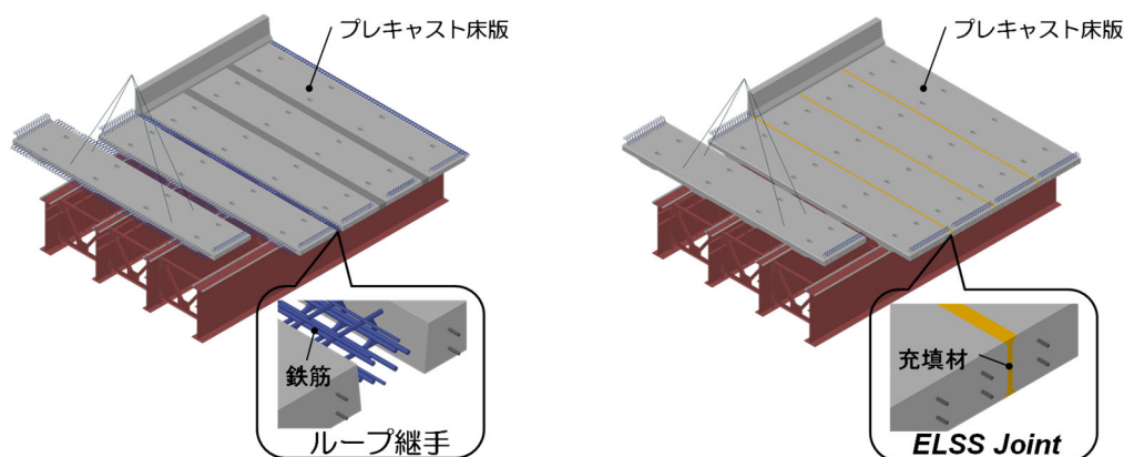
【従来のループ継手（左）と開発した継手構造（右）の構造概要】
