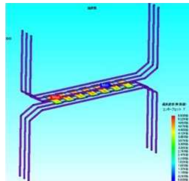
▲『SolidWorks(ソリッドワークス)』で3次元設計、『JMAG(ジェイマグ)』で電磁界・熱流体解析
