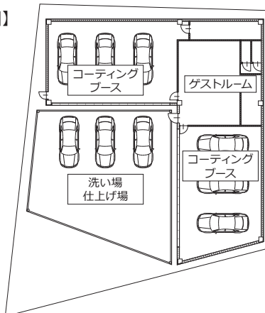
【店舗平面図】
