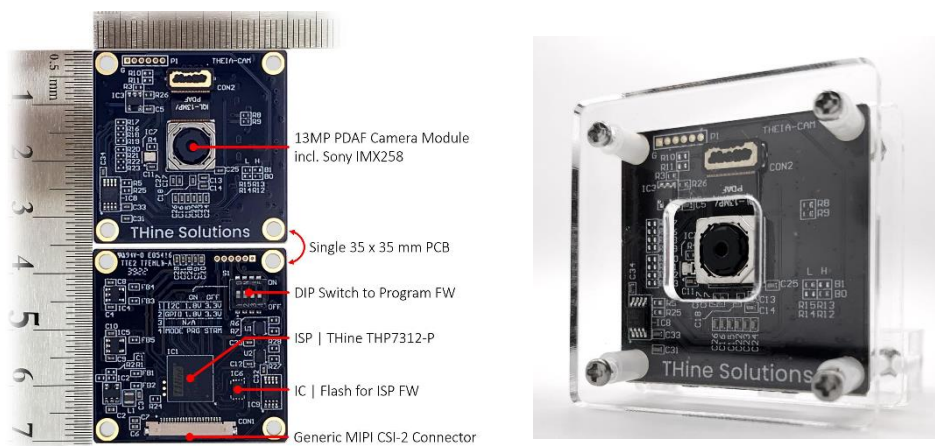
THSCJ101 の写真
